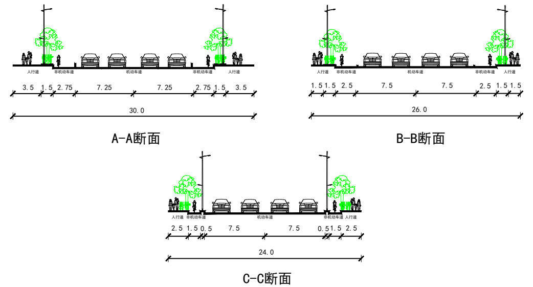
道路断面图
