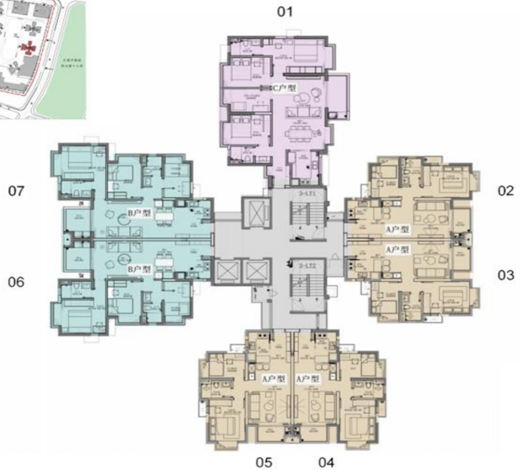
3栋标准层平面图 (注：图中编号为房号)
