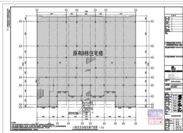
首层加装平面图
