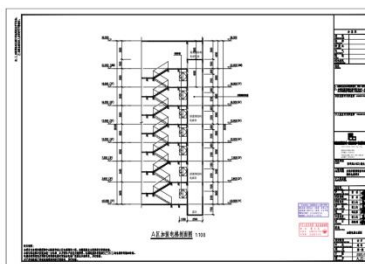
加装电梯剖面图
